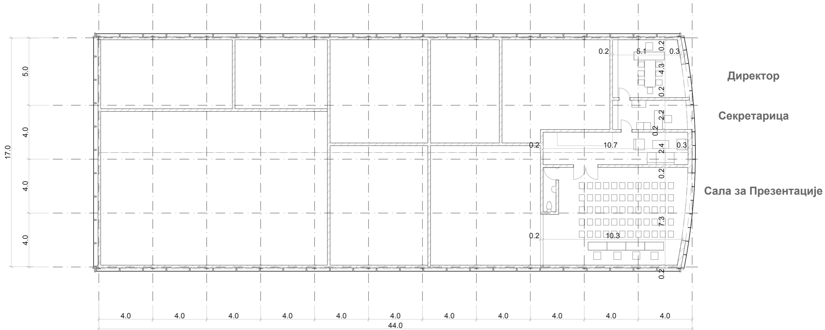
Основа Спрата P 1:200
